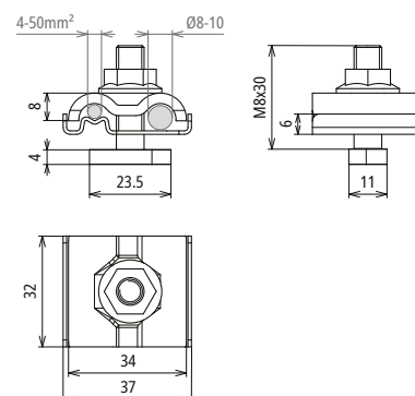
Maßbild UEK 8.10 AQ4 50 HKSM8 V2A
