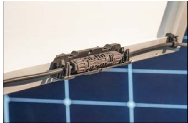
Einfache Handmontage auf Kanten von 1,0–3,0 mm – ideal für PV-Installationen.
